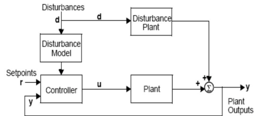
Fig.12: Controlador GPC, con perturbaciones.
