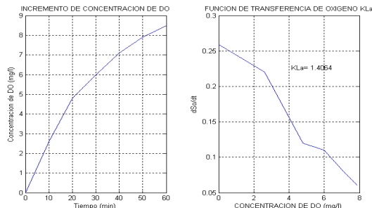
Fig.5: Izquierda: Aumento concentración de DO. Derecha: K_{La} = 1.4064 , obtenido como la pendiente de dS_o/dt con respecto S_o .
